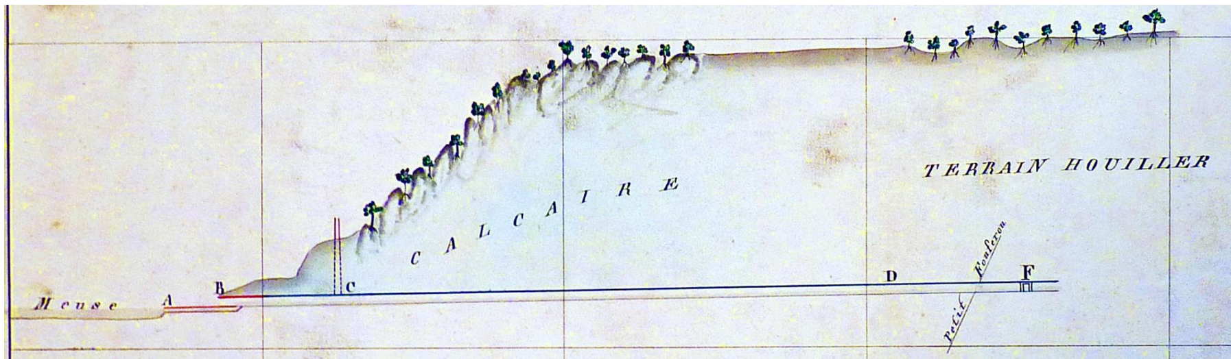
Coupe perpendiculaire à la galerie d'écoulement, donc en travers bancs passant par le Vieux Murguet « F ». La couche de charbon « Petit Fouferou », sans doute aussi appelée par ailleurs « Petite veine », est la première couche de charbon exploitable juste après le calcaire formant la falaise et avant « Fouferou ».
