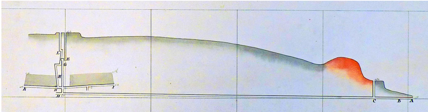
Coupe suivant la direction de la couche Fouferou montrant deux panneaux exploités de part et d'autre des puits du Vieux Murguet ainsi que de la galerie d'écoulement DA vers Bende. En orange, les dépôts de schistes brûlés provenant de la fabrique d'alun située en Bende.
